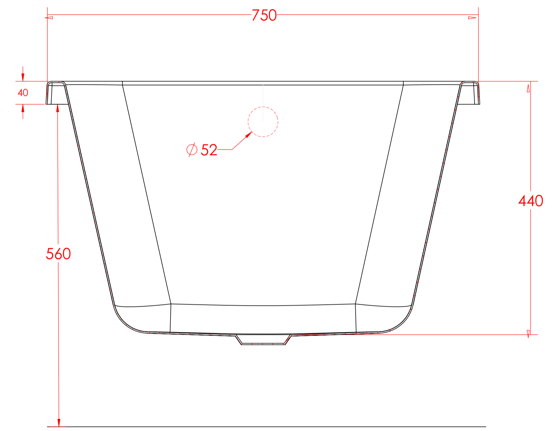
SECTION A-A SCALE 1 : 4
