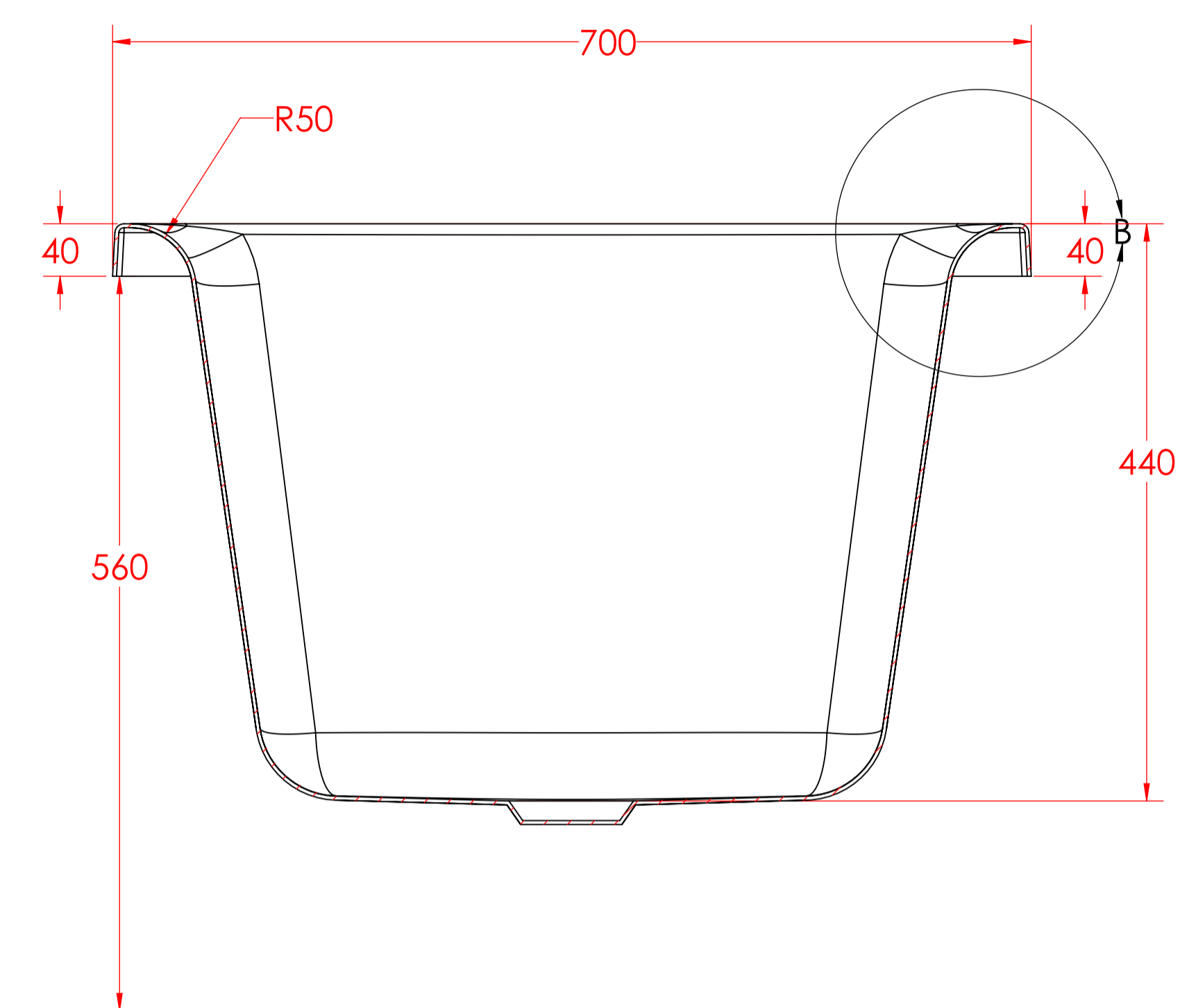
SECTION A-A SCALE 1 : 4
