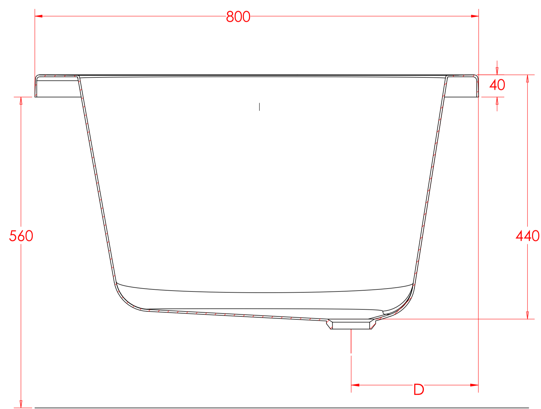
SECTION G-G SCALE 1 : 4
